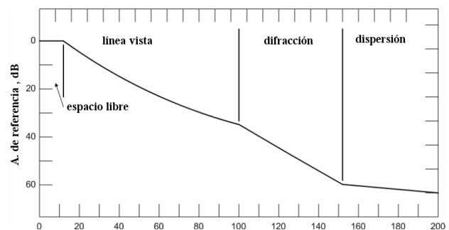
Figura 3: Atenuación de referencia vs. distancia.[4]
