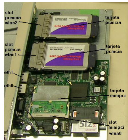
Figura 2: Placa Soekris con tres interfaces inalámbricas.
