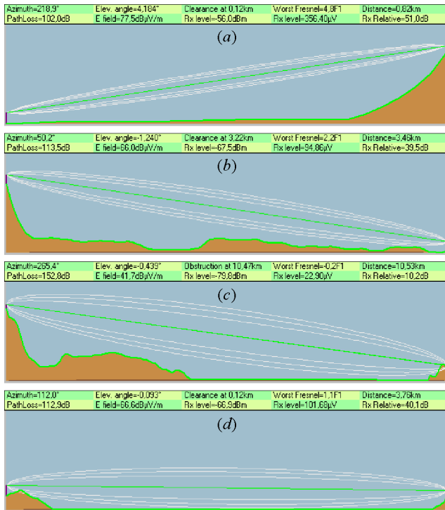
Figura 6: Perfil topográfico de los enlaces implementados. (a) Municipalidad – Repetidor; (b) Repetidor – Sta. Agueda; (c) Repetidor - Sotomó; (d) Sotomó – Yates.
