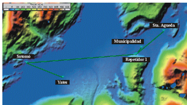
Figura 4: Proyección de los enlaces, vista SRTM3.
